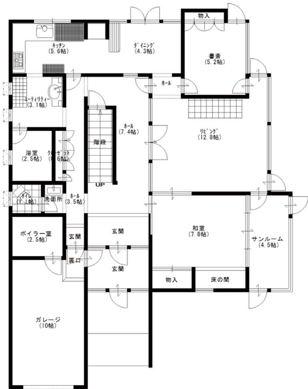
1F 平面図
